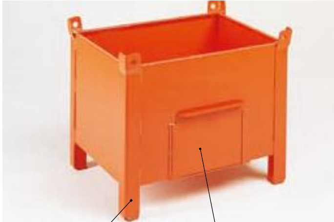
PIEDE SCATOLATO BOXED FOOT TRAMOGGIA CON PORTA A GHILOTTINA HOPPER WITH GUILLOTINE GATE
