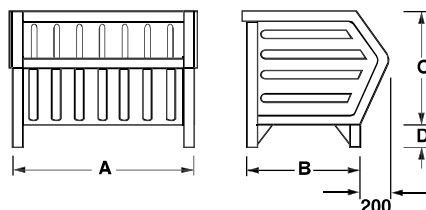
SU RICHIESTA SLITTA LATO CORTO SKID ON SHORT SIDE AVAILABLE ON REQUEST
