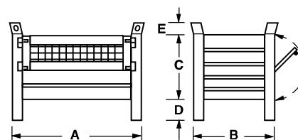
PIEDE SCATOLATO BOXED FOOT
