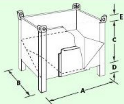
Tramoggia con porta a ghigliottina e piano interno inclinato Hopper with guillotine gate and tilted internal surface
