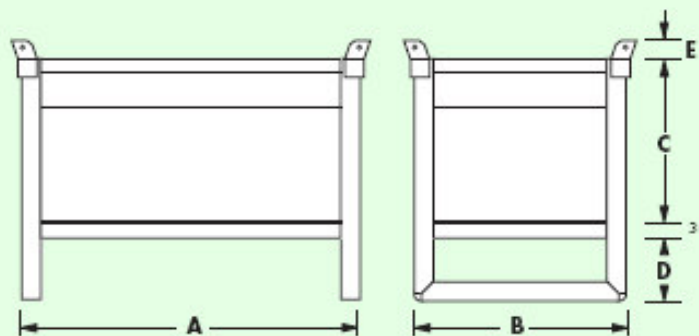
Pareti in lamiera liscia, nessun bordo interno, per facilitare lo scarico del materiale Walls in plain sheet, no inside edge, to facilitate unloading of the material
