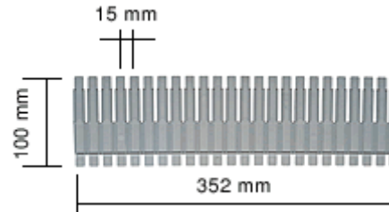
MODELLO UNITÀ D'IMBALLO Divit 400 50
