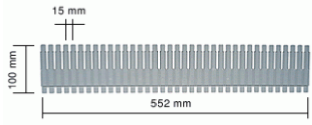
MODELLO UNITÀ D'IMBALLO Divit 600 40
